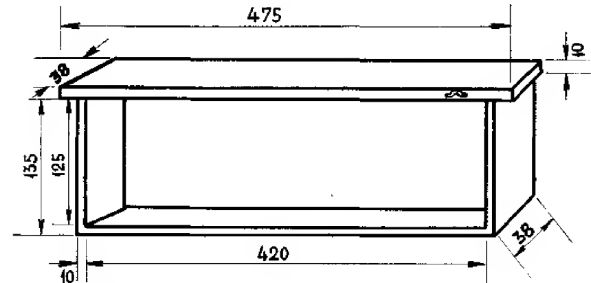
Медишни широки полуоквир за преуређене Дадан-Блатове кошнице (Мере изражене у mm)
